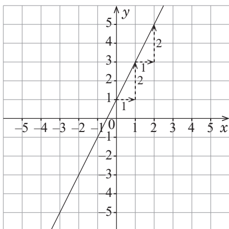
Gráfica \ell y = 2x + 1
