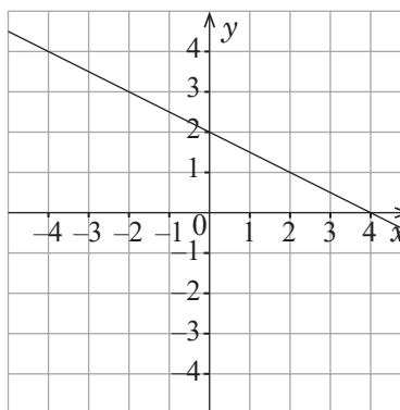
Gráfica m y = -\frac{1}{2}x + 2
