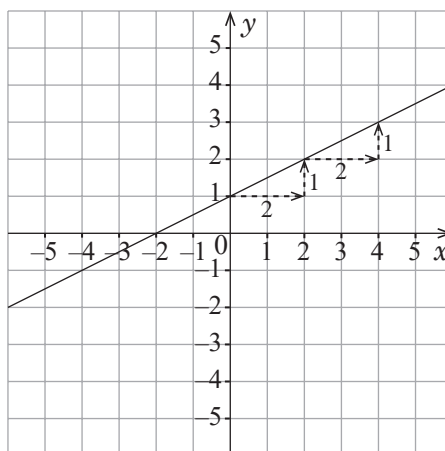
Gráfica m y = \frac{1}{2}x + 1
