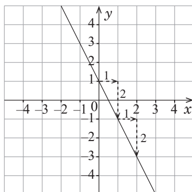
Gráfica \ell y = -2x + 1
